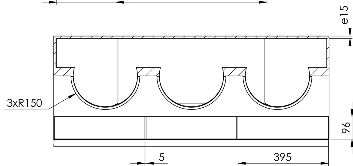
SECCIÓN E-E ESCALA 1 : 10
